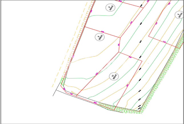
PLAN FONCIER DU LOT Echelle : 1/500
